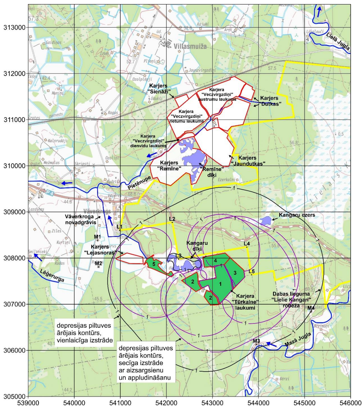
3.8. att. Ūdens līmeņu depresijas piltuvju salīdzinājums, slānim D3dg#
