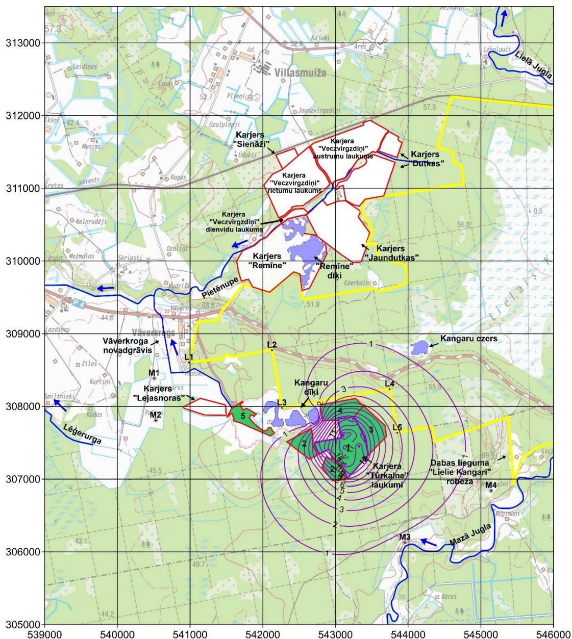
3.3. att. Depresijas piltuve karjeram Tūrkalne, slānī D3dg#, pirmais laukums [m]
