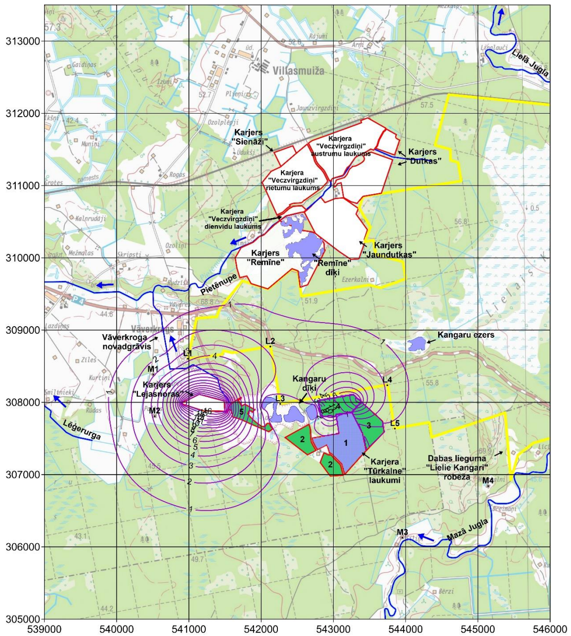
4.10. att. Depresijas piltuve atsūknējot Tūrkalne un Lejasnoras, slānī D3dg# , 4 etaps [m]
