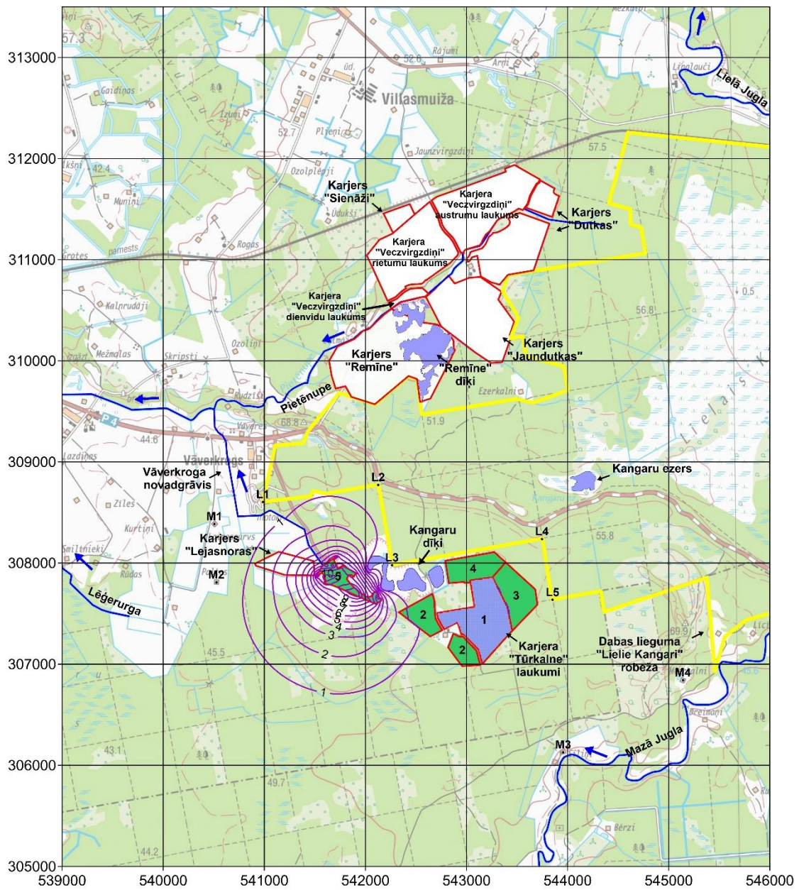
3.7. att. Depresijas piltuve karjeram Türkalne, slānī D3dg#, piektais laukums [m]
