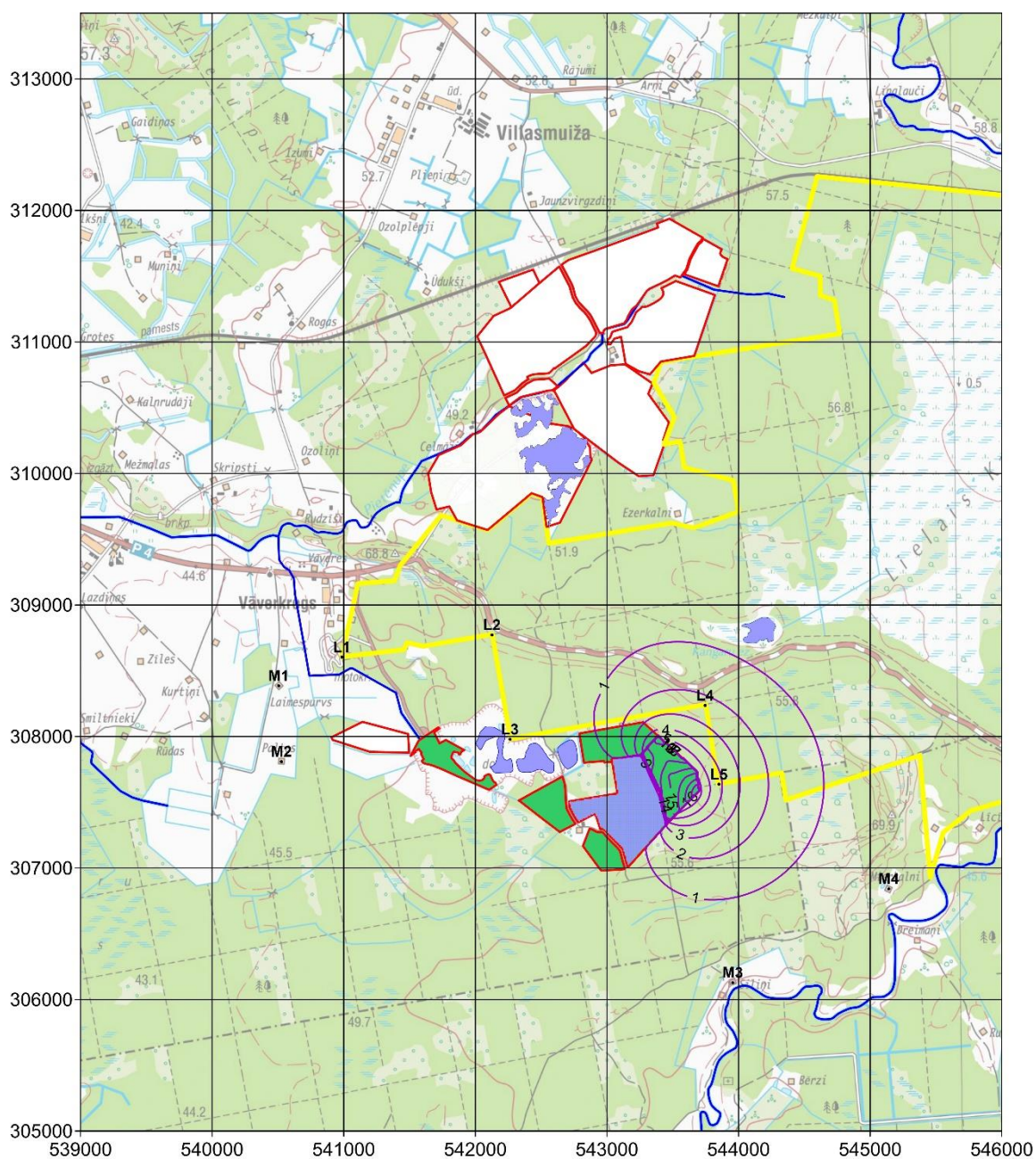
5.10 att. Depresijas piltuves izmaiņas, Tūrkalne trešais etaps ar pastiprinātu ārsienu, slānī D3dg#, esošā situācijā [m]
