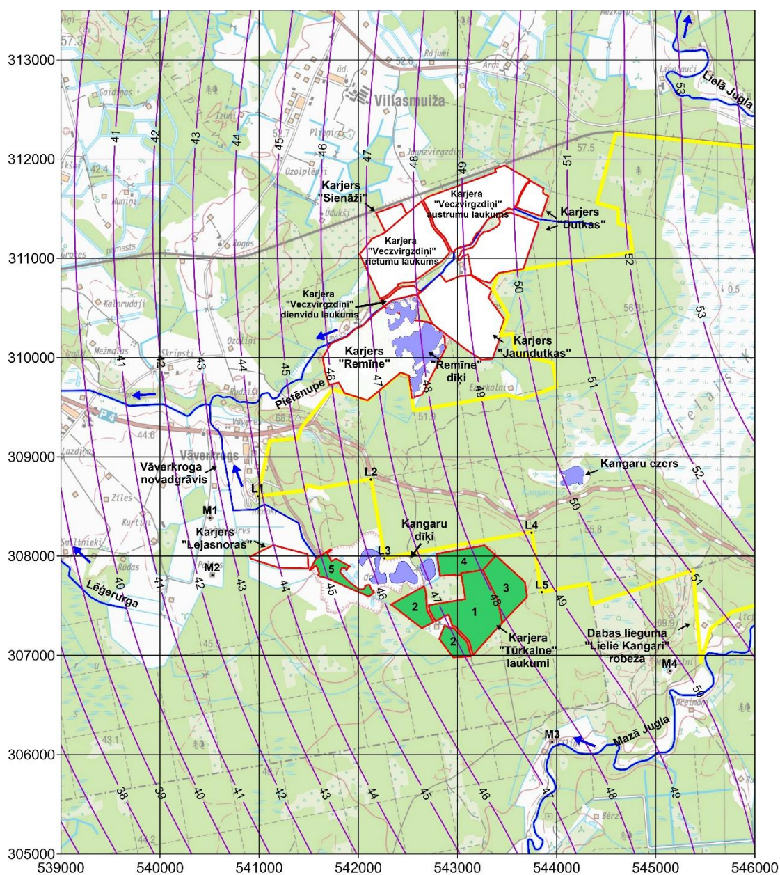
2.4. att. Ūdens līmeņu izolīnijas slānī D3pl [m vjl]
