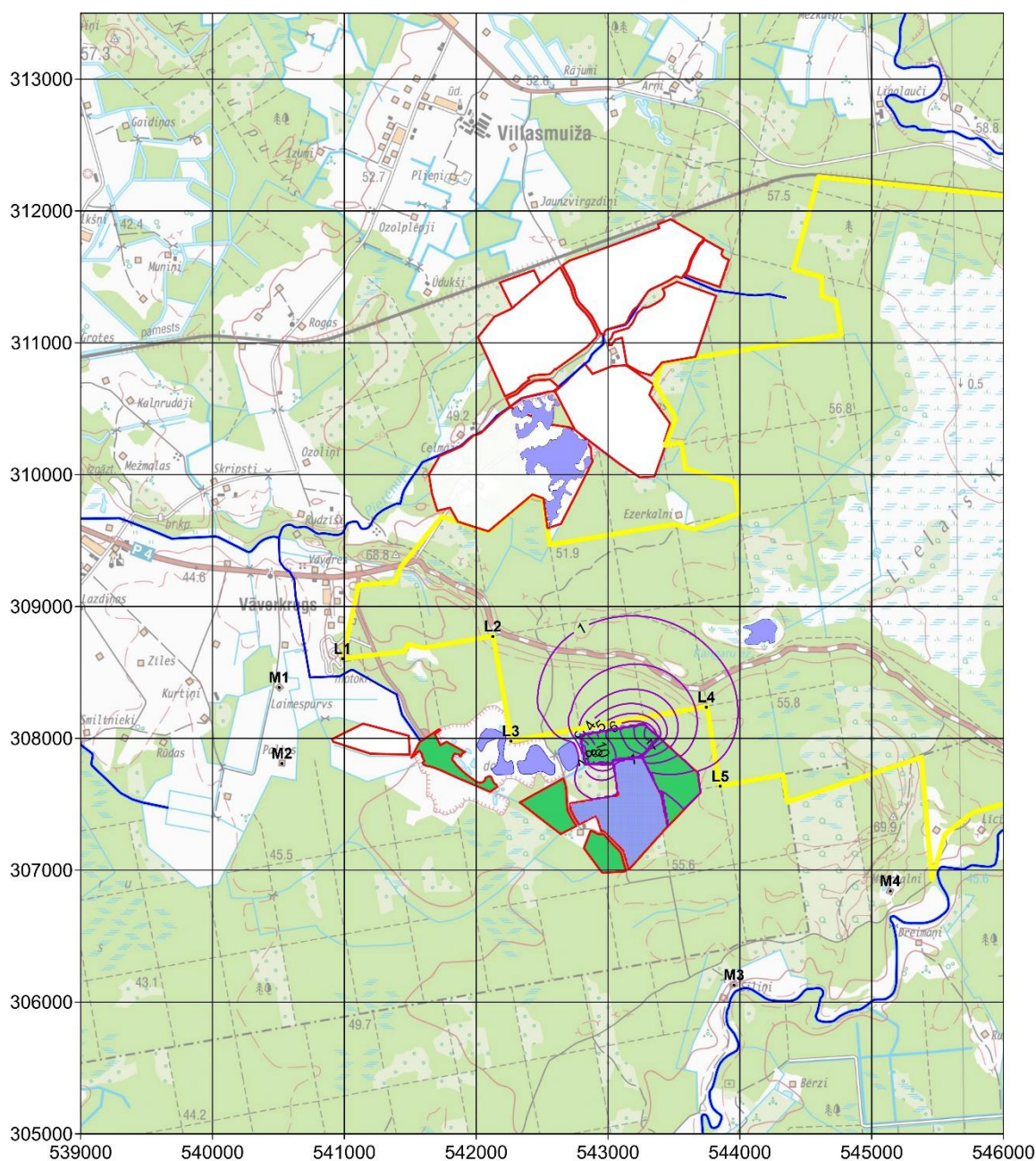
5.12 att. Depresijas piltuves izmaiņas, Tūrkalne ceturtais etaps, slānī D3dg#, esošā situācijā [m]
