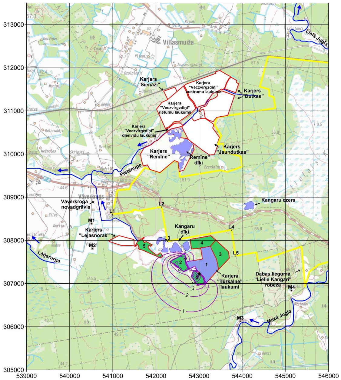
4.7. att. Depresijas piltuves izmaiņas atsūknējot Tūrkalne un Lejasnoras, slānī D3dg#, 2 etaps [m]
