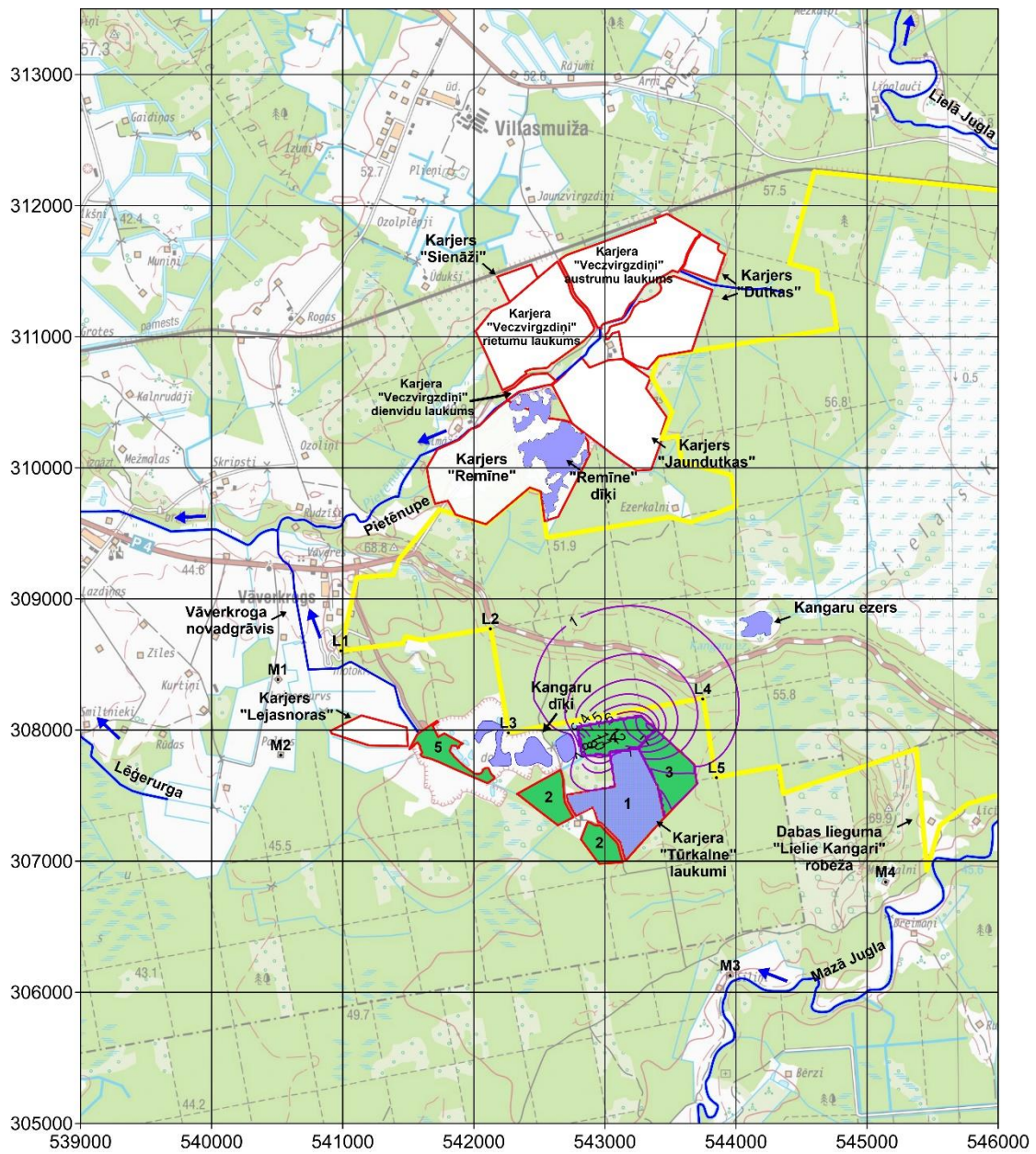
4.11. att. Depresijas piltuves izmaiņas atsūknējot Tūrkalne un Lejasnoras, slānī D3dg#, 4 etaps [m]
