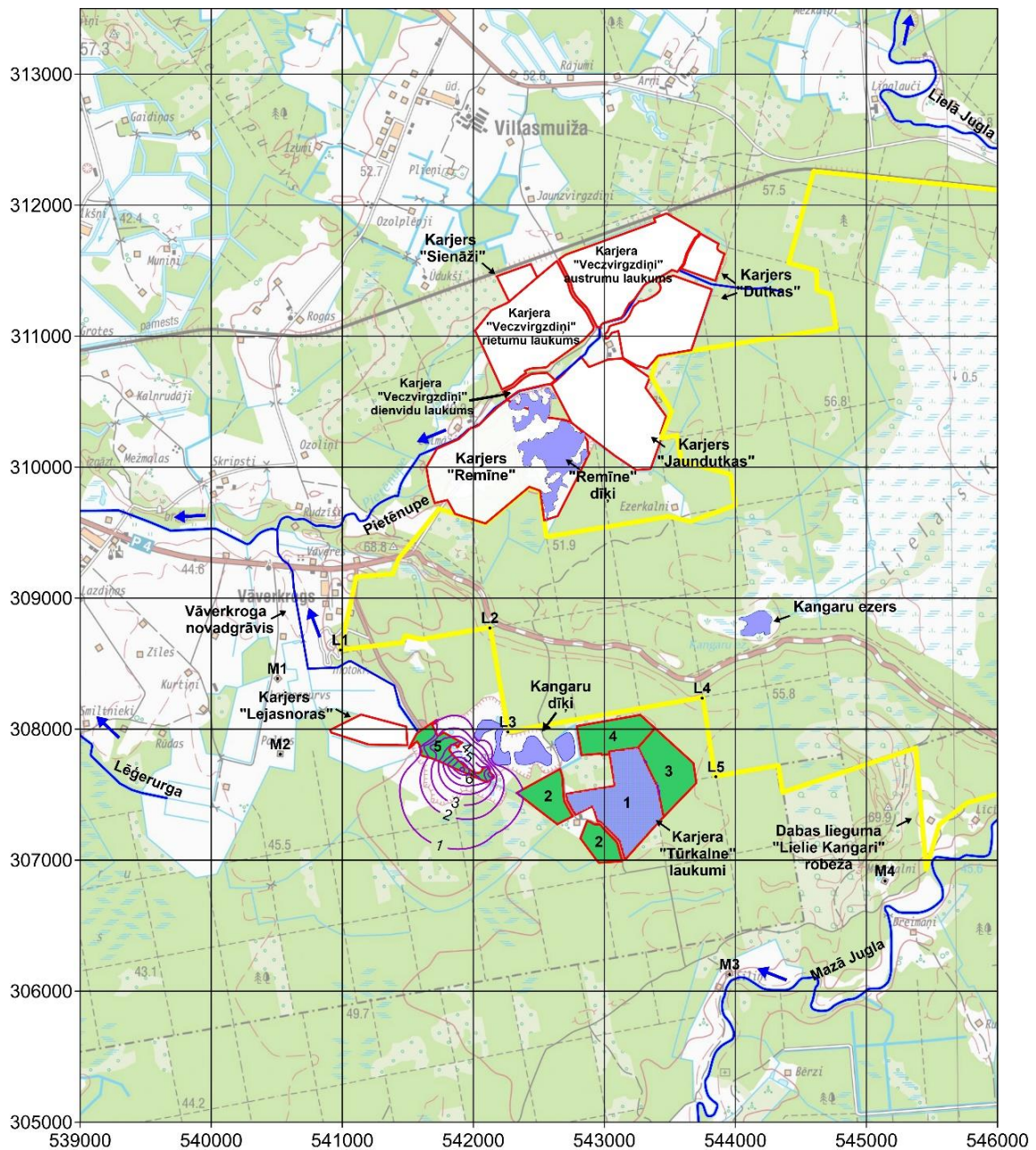
4.13. att. Depresijas piltuves izmaiņas atsūknējot Tūrkalne un Lejasnoras, slānī D3dg\# , 5 etaps [m]
