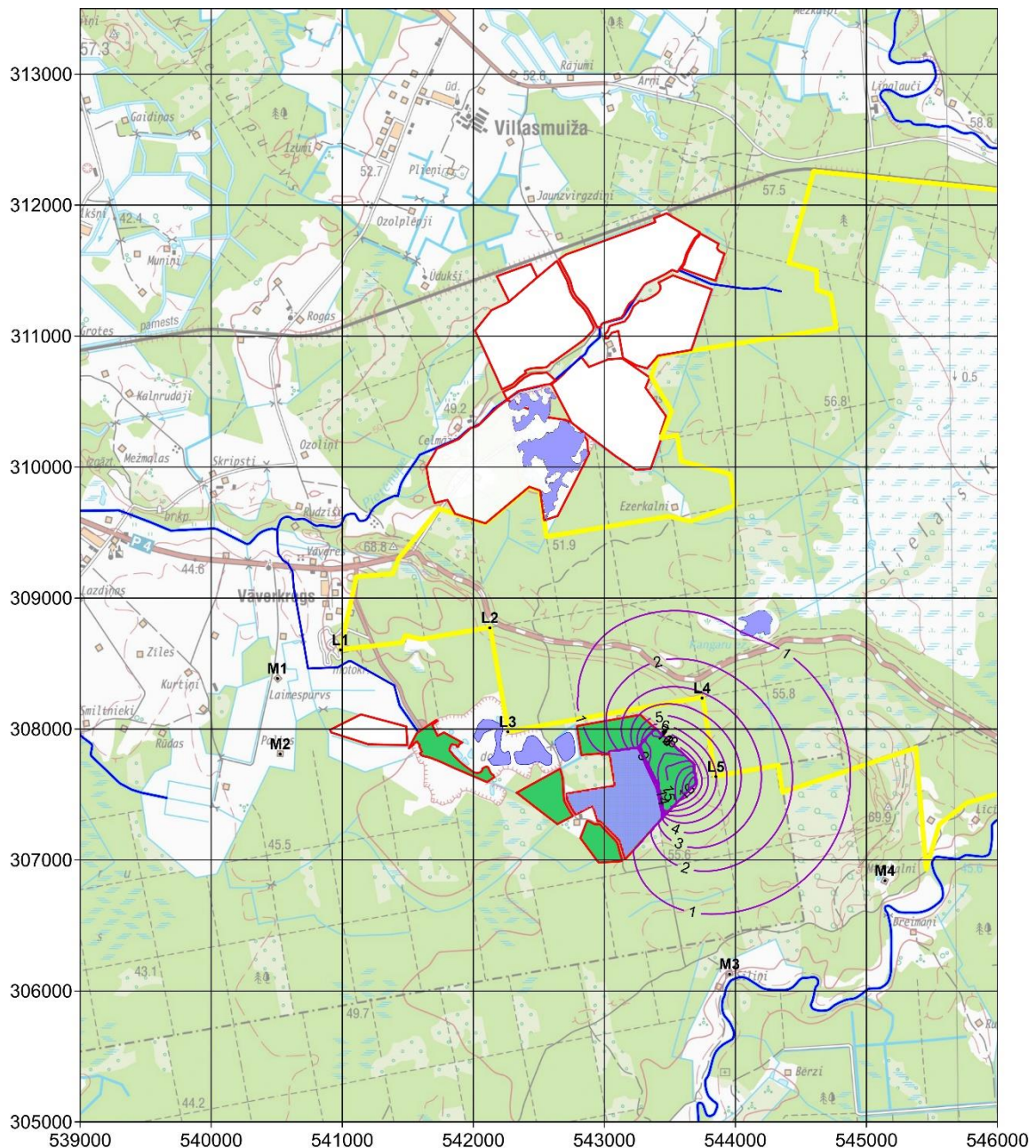
5.9. att. Depresijas piltuves izmaiņas, Tūrkalne trešais etaps slānī D3dg# , esošā situācijā [m]
