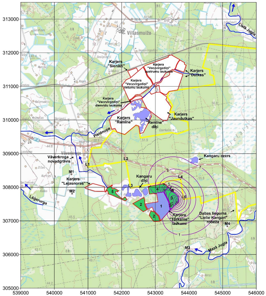
3.5. att. Depresijas piltuve karjeram Tūrkalne, slānī D3dg#, trešais laukums [m]
