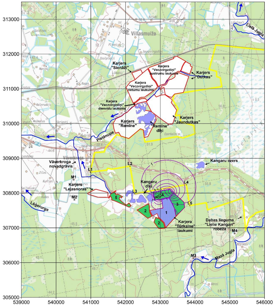
3.6. att. Depresijas piltuve karjeram Tūrkalne, slānī D3dg#, ceturtais laukums [m]
