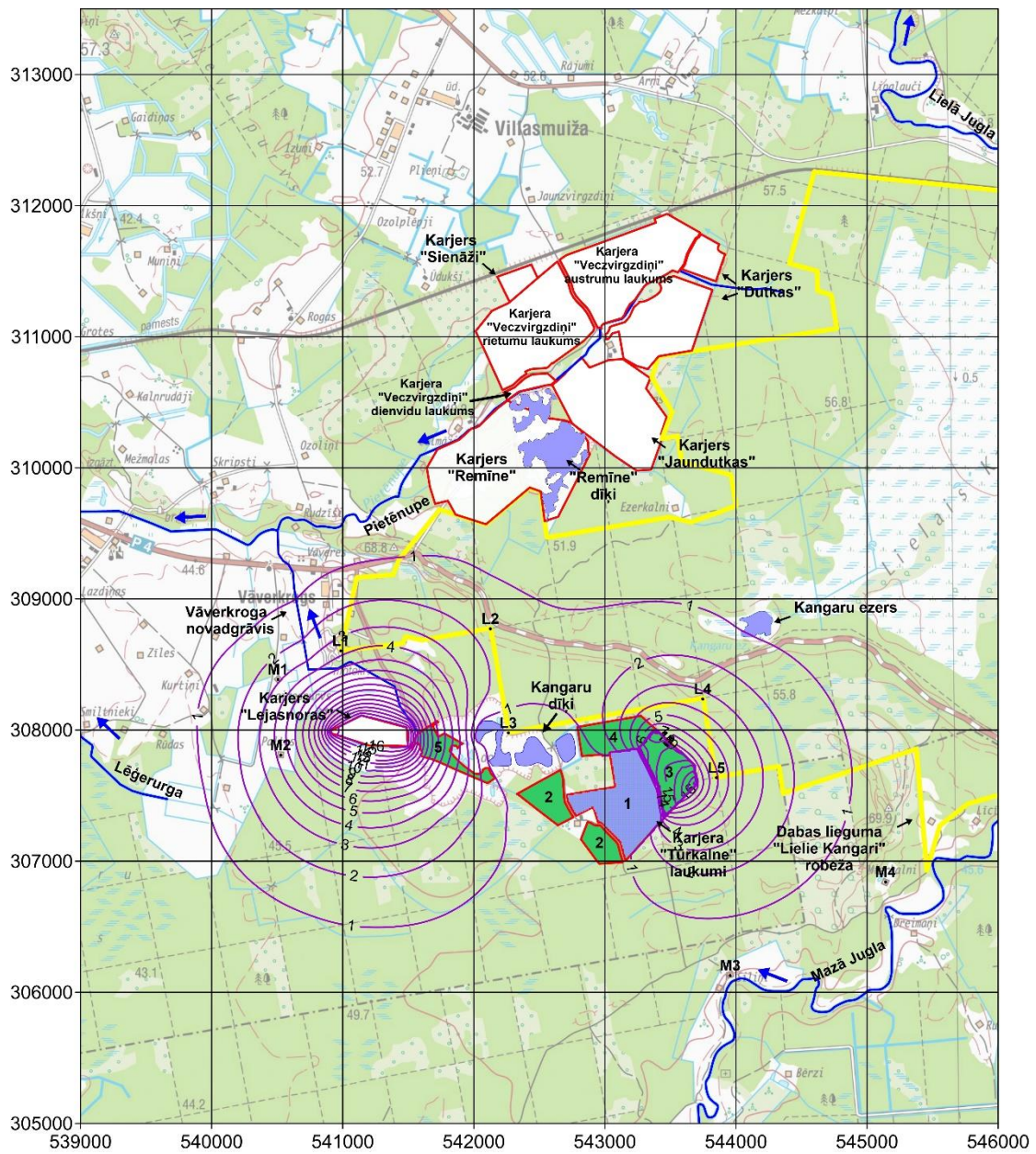
4.8. att. Depresijas piltuve atsūknējot Tūrkalne un Lejasnoras, slānī D3dg#, 3 etaps [m]
