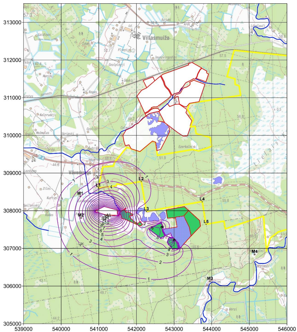
4.6. att. Depresijas piltuve atsūknējot Tūrkalne un Lejasnoras, slānī D3dg#, 2 etaps [m]
