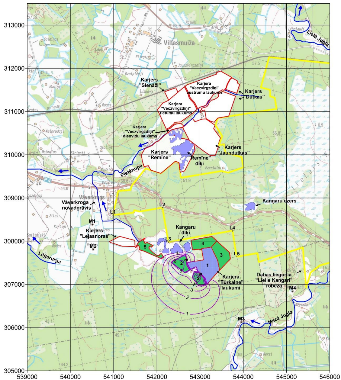
3.4. att. Depresijas piltuve karjeram Tūrkalne, slānī D3dg#, otrais laukums [m]
