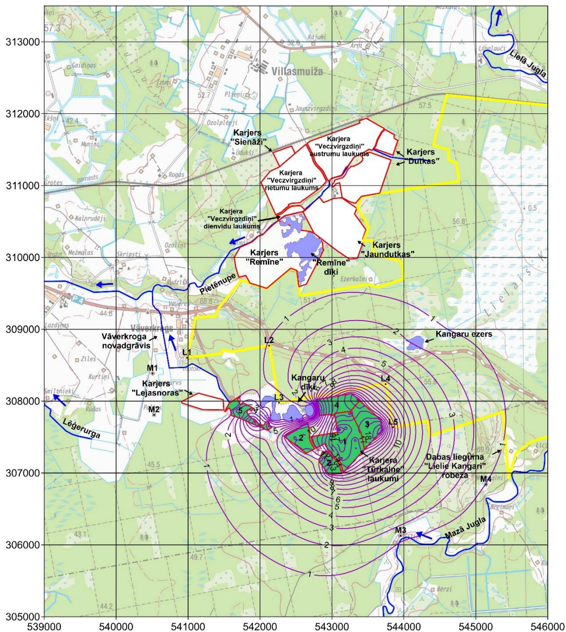
4.3. att. Tūrkalne depresijas piltuves izmaiņas, slānī D3dg#, visi laukumi [m]
