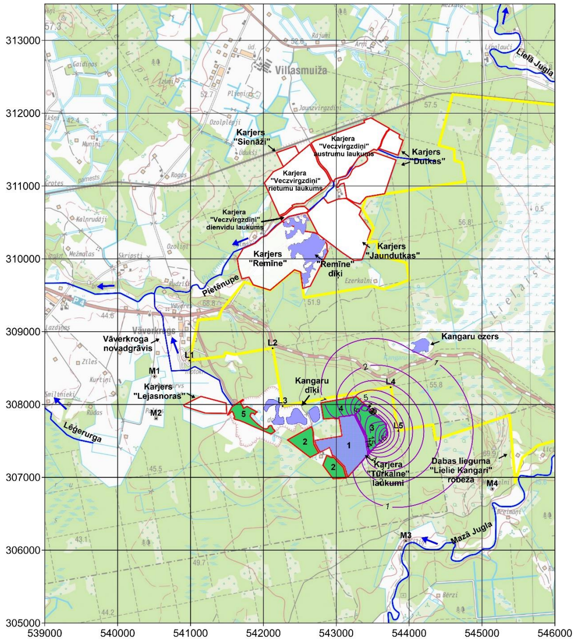
4.9. att. Depresijas piltuves izmaiņas atsūknējot Tūrkalne un Lejasnoras, slāņī D3dg#, 3 etaps [m]
