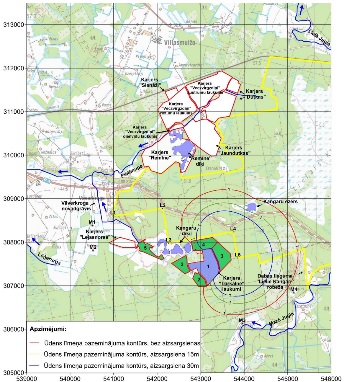
5.11. att. Depresijas piltuves izmaiņas, Tūrkalne trešais etaps, slānī D3dg#, izstrādes variantu salīdzinājums[m]
