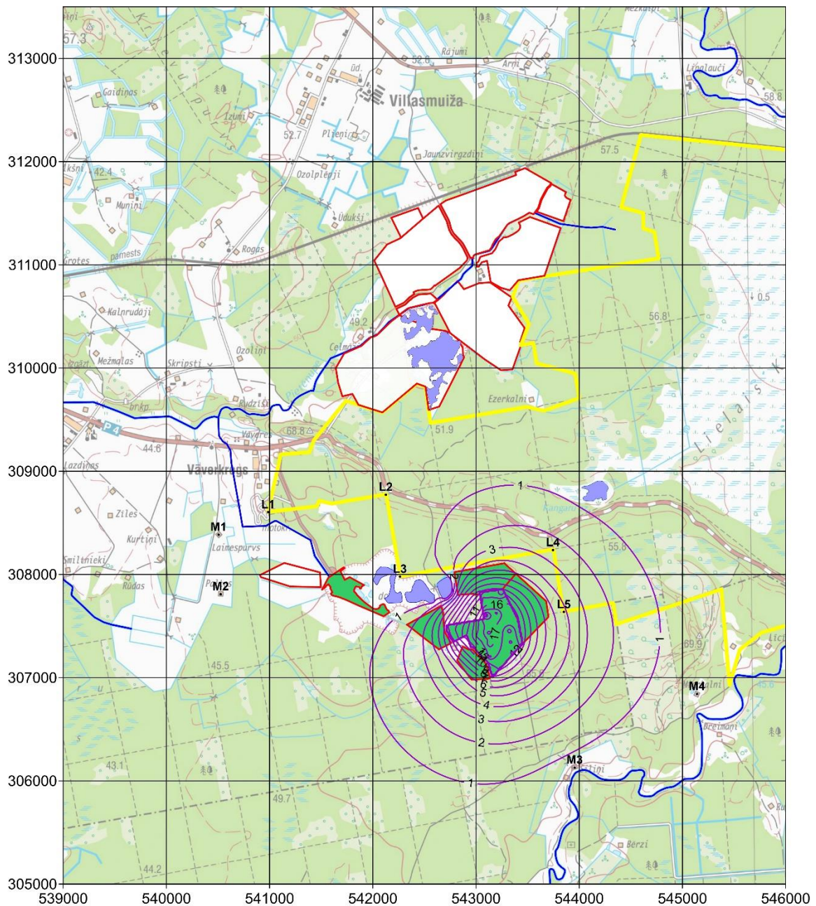
5.6. att. Depresijas piltuves izmaiņas, Tūrkalne pirmais etaps slānī D3dg# , esošā situācijā [m]
